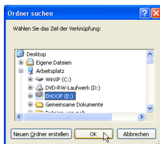
Bild 4: Verzeichnisbaum
